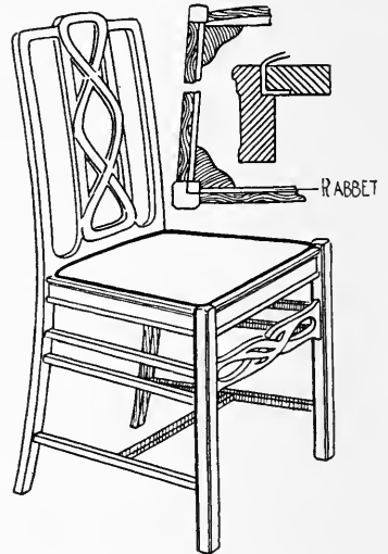
FIG. 481. SLIP-SEAT.
